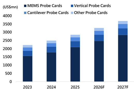
圖 7：探針卡產值將以 CAGR 12%成長至 2027 年
